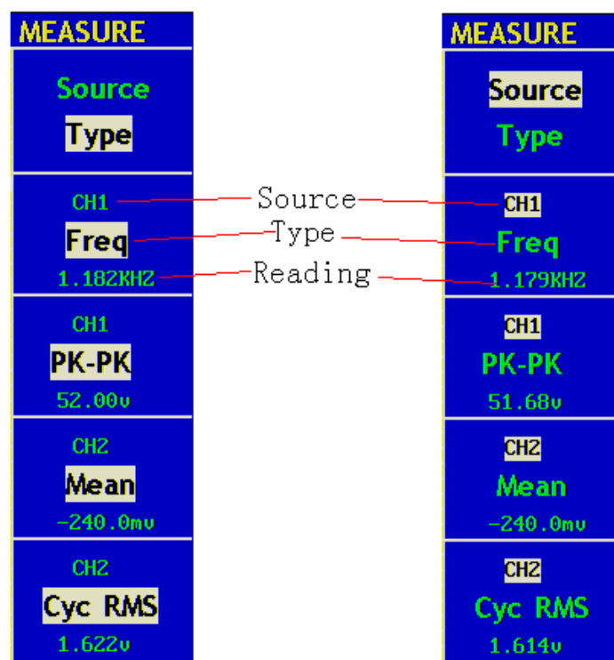
Fig.57 Measure Menu
